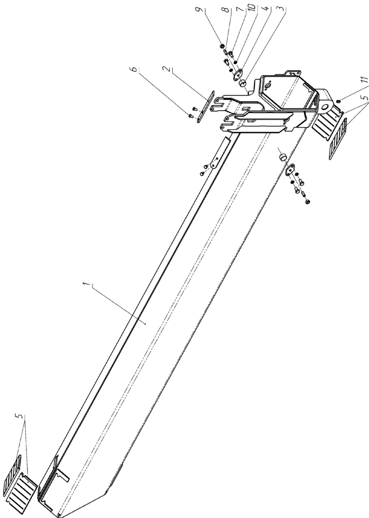
Рисунок 10.1 – Секция телескопирования вторая
