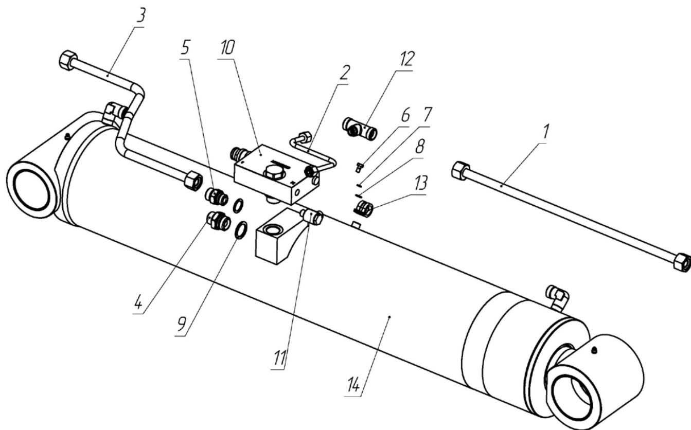
Рисунок 8.2 – Гидроцилиндр подъёма второй стрелы (для АНТ22-2)
