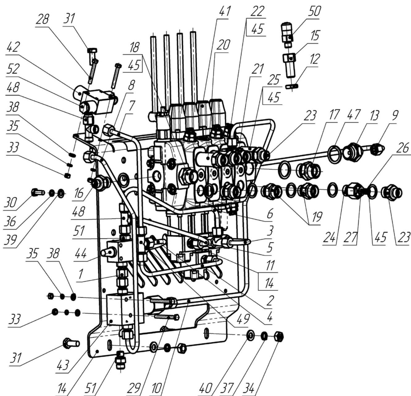
Рисунок 20.1 – Обвязка гидрораспределителя
