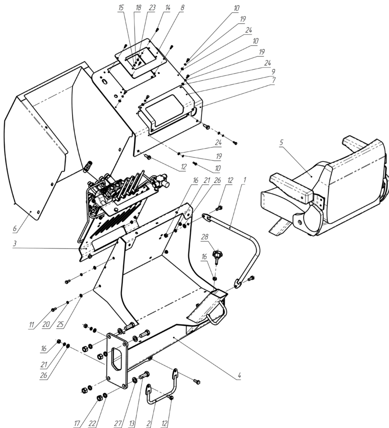
Рисунок 19.1 – Пульт верхнего управления
