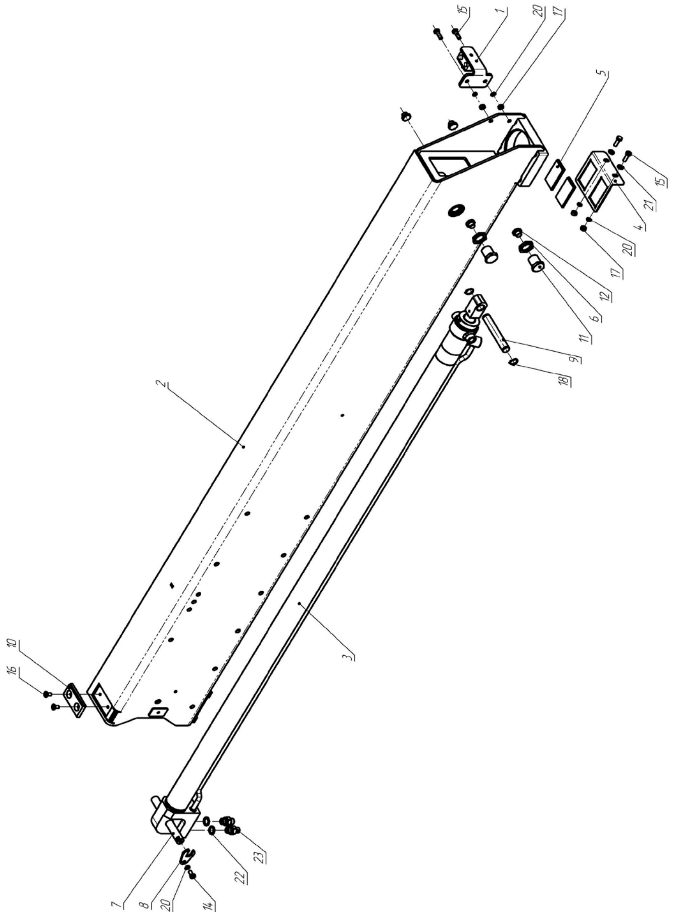
Рисунок 17.1 – Балка выносная
