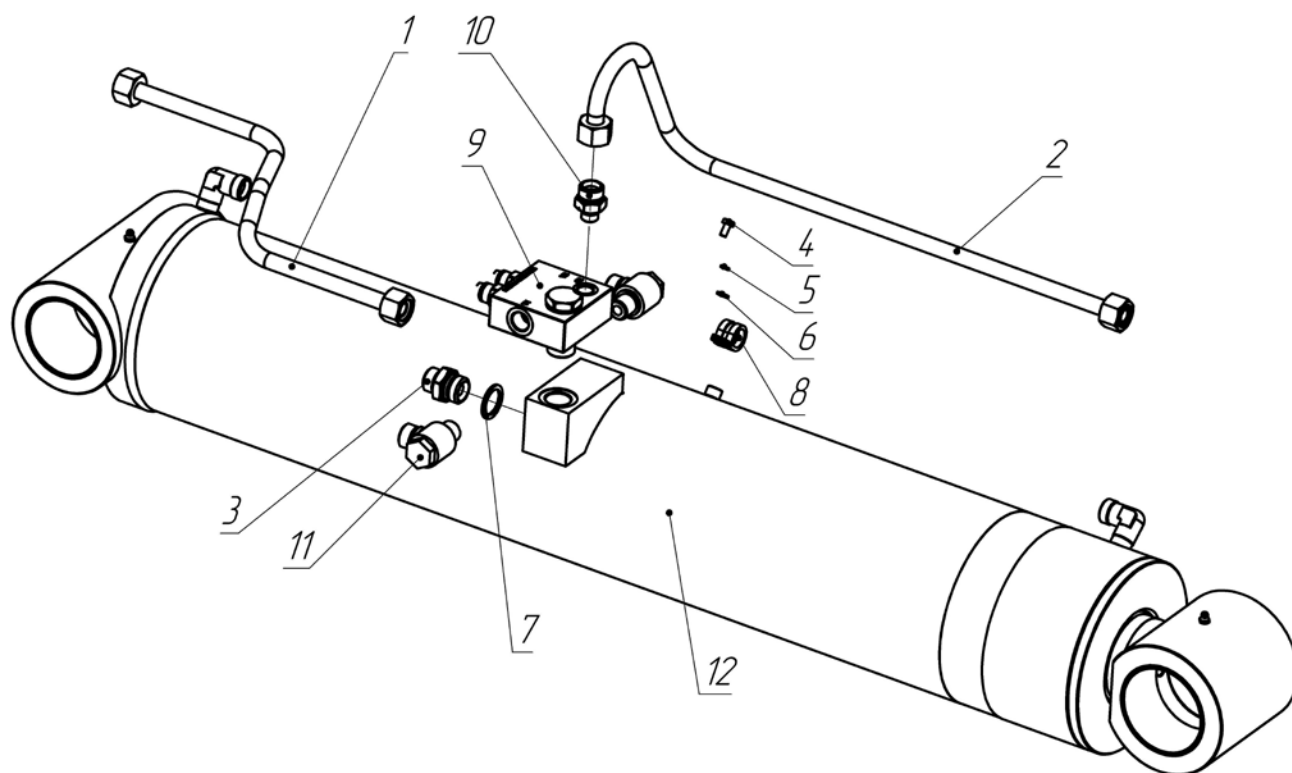
Рисунок 8.1 – Гидроцилиндр подъёма второй стрелы (для АНТ22-4, АНТ22-3)
