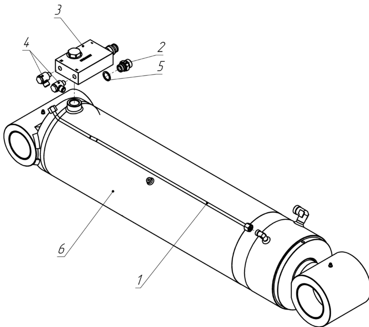
Рисунок 5.1 – Гидроцилиндр подъёма первой стрелы
