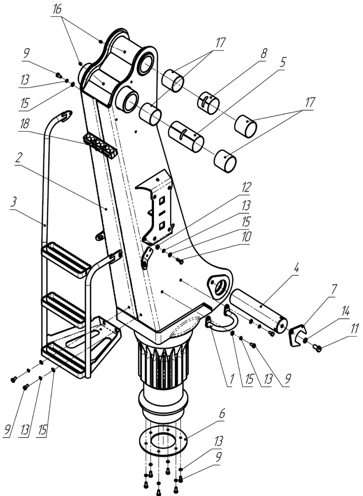
Рисунок 3.1 – Колонна
