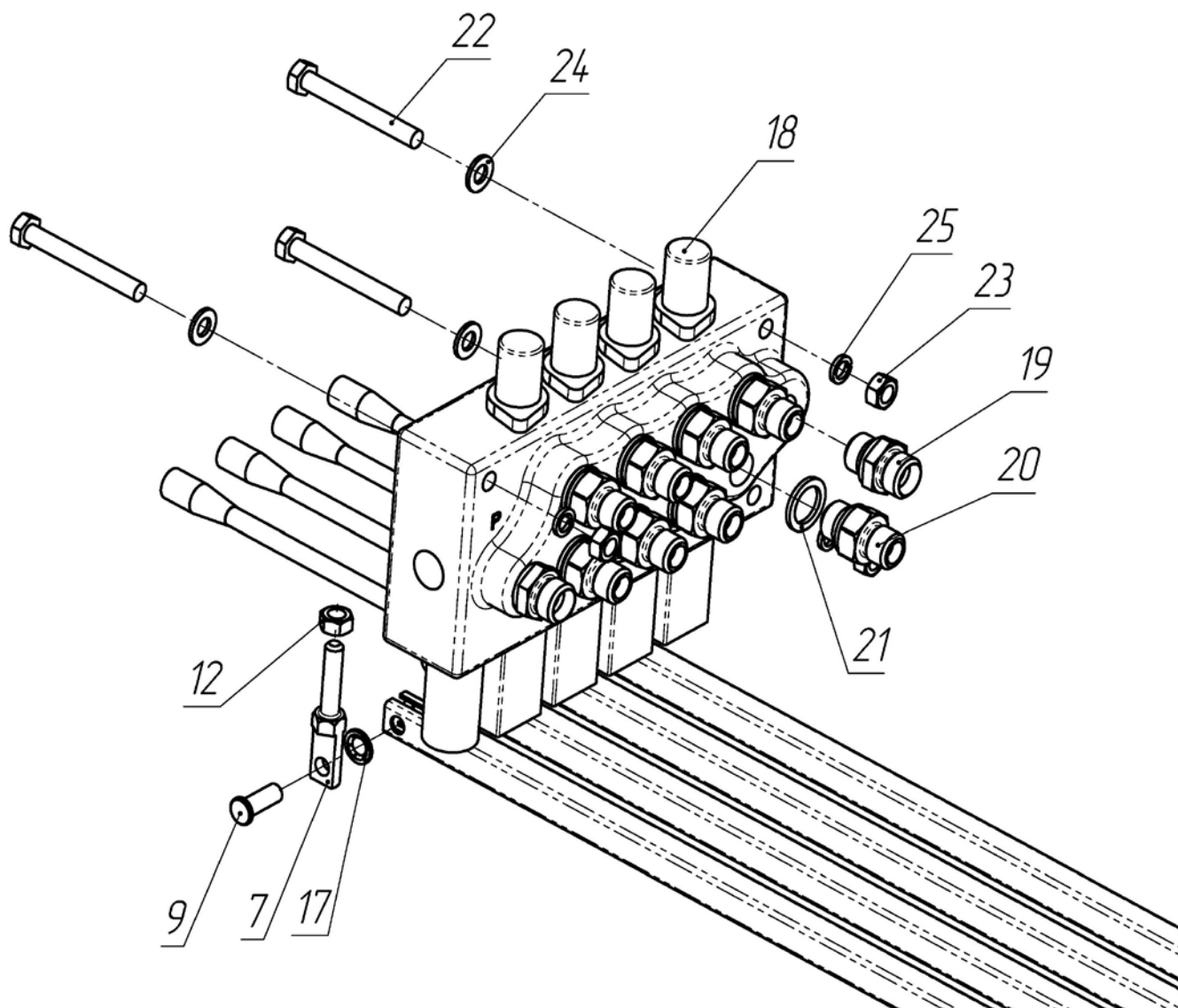
Рисунок 21.3 – Опора в сборе
