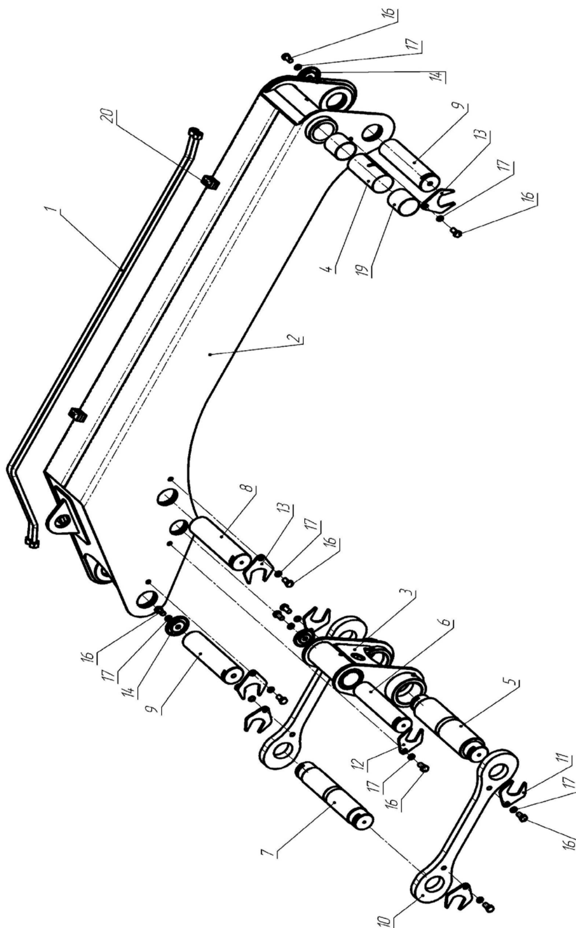
Рисунок 4.1 – Стрела первая
